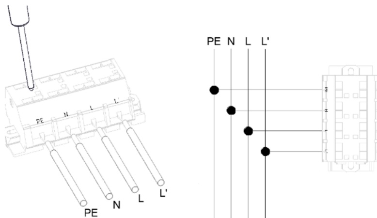
Rysunek 3. Możliwe schematy podłączenia opraw serii PrimeLine
