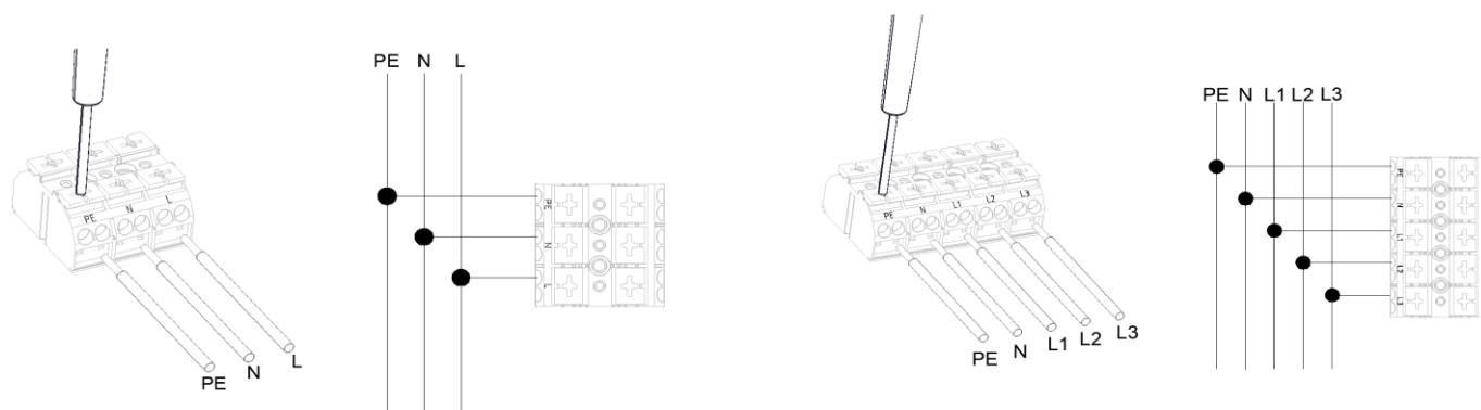
Rysunek 5. Możliwe schematy podłączenia opraw serii PrimeLine
