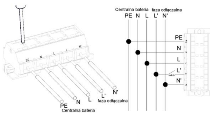
Schemat podłączenia oprawy oświetleniowej z wbudowanym modulem CBY-M1
