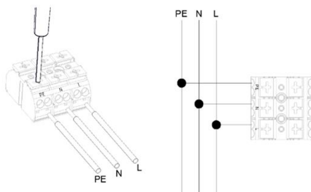
Schemat podłączenia oprawy oświetleniowej z wbudowanym modulem CBX-M1
